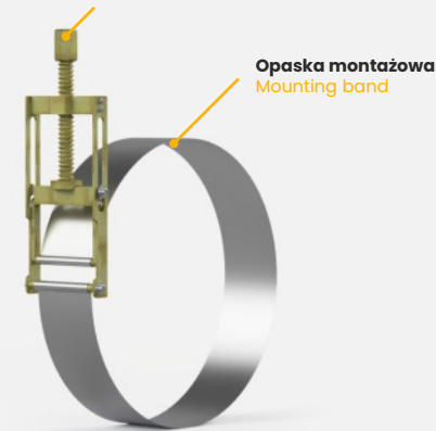
Klamra śrubowa dla średnic Ø110 – Ø200 mm Screw locker for diameter Ø110 – Ø200 mm
